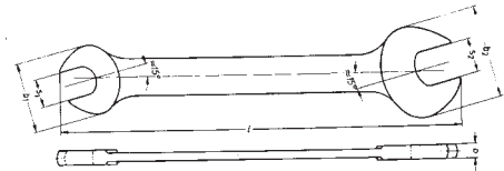
Technische Abbildung Nr.3 lt. DIN 3110 Technical Picture 3
