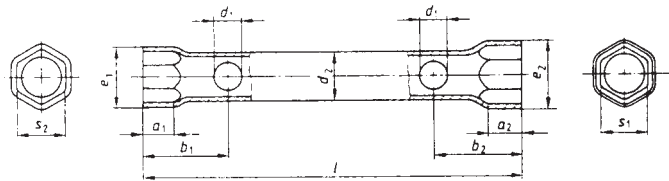
Technische Abbildung Nr.7 lt. DIN 896 Technical Picture 7
