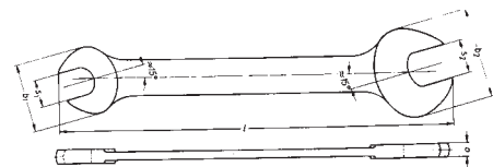
Technische Abbildung Nr.2 lt. DIN 895 Technical Picture 2
