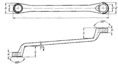
Technische Abbildung Nr.6 lt. DIN 838 Technical Picture 6
