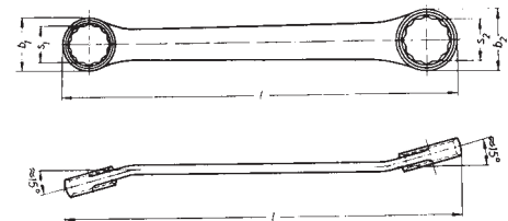
Technische Abbildung Nr.5 lt. DIN 837 A Technical Picture 5
