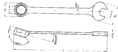
Technische Abbildung Nr.4 lt. DIN 3113 A Technical Picture 4
