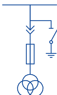
Трансформатор напряжения + заземление сб. шин
