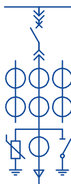
Отходящая линия
