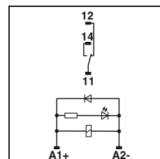
Катушка постоян. тока
