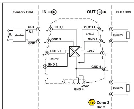
конфигурируемый, с двумя выходными сигналами тока
