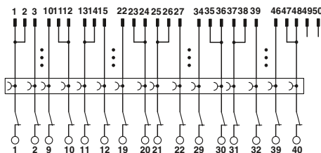
Схема подключения FLKM 50/KDS3-MT/PPA/S7-300
