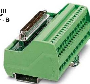
37 полюсов, с винтовыми зажимами или с зажимами Push-in
