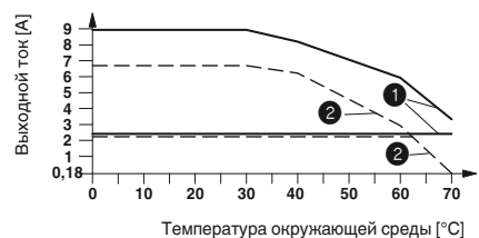
Кривая изменения характеристик ELR H5-IES-SC-24DC/500AC-2 и ELR H5-IES-SC-24DC/500AC-9 Продолжительность включения 100 %
