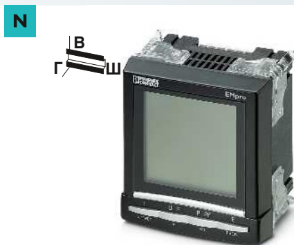
Измеряемое напряжение до 500 В переменного тока, с возможностью расширения посредством интерфейса RS-485
