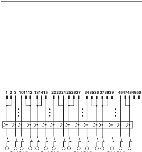
Схема подключения FLKM 50/KDS3-MT/PPA/PLC
