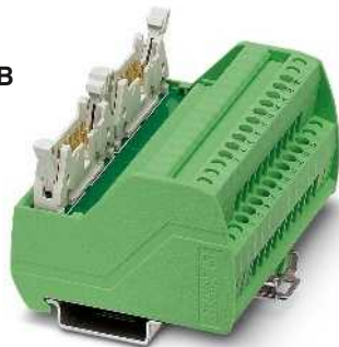
Пассивные интерфейсные модули для SIMATIC® S7-300 с винтовыми зажимами
