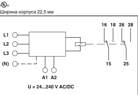
Реле контроля пониженного напряжения и фаз на 400 или 230 В
