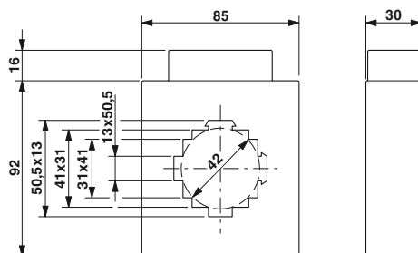
Шинный трансформатор тока с возможностью дополнительной поверки
