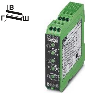
Многофункциональное реле времени, с двумя настройками времени
