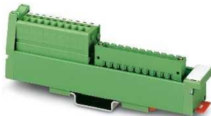
10- и 18-полюсн. с винтовыми зажимами
