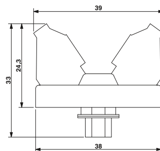
Чертеж DFLK-D...SUB
