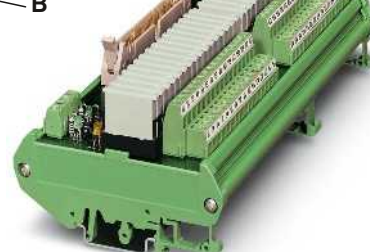
Базовый модуль вывода с 32 миниатюрными реле, 1 замыкающих контакта
