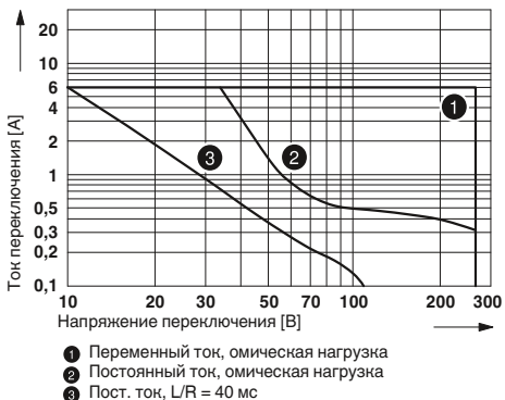
Электрическая мощность отключения для PLC...21HC для высоких токов длительной нагрузки
