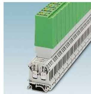
Силовые полупроводниковые реле с выходом 400 В пер. тока / 3 А
