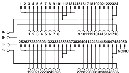
Схема подключения FLKM 50-PA-AB/1756/IN/EXTC
