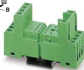
2/2-ярусная конструкция с винтовыми зажимами
