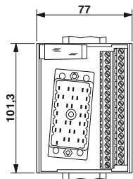
Чертеж UMK-EC90/32/EX-XUL
