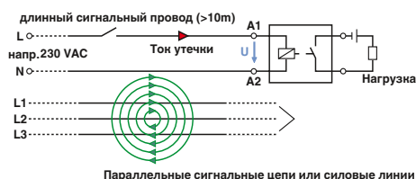
Возникновение паразитных сигналов: Вариант 2: длинные сигнальные провода
