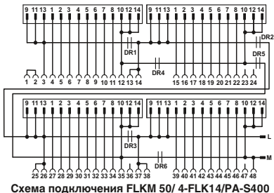
Схема подключения FLKM 50/ 4-FLK14/PA-S400
