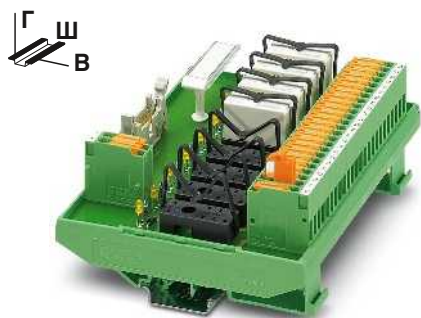
Модуль вывода для 8 мини-реле с клеммами с размыкателями, 1 переключающий контакт
