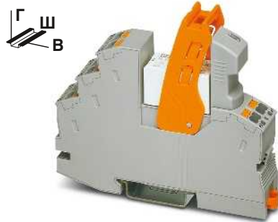
Релейный модуль RIF-1 с реле с 2 переключающими контактами
