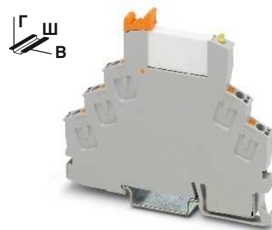
Релейный модуль RIF-0 с реле с 1 переключающим контактом
