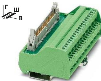
Пассивные интерфейсные модули для ввода-вывода со специфической маркировкой и винтовым зажимом
