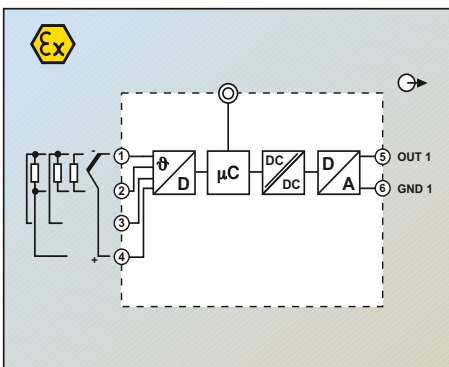
Блок-схема MCR-FL-T-LP-I-EX
