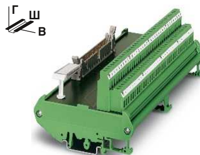
Пассивные интерфейсные модули с винтовыми зажимами
