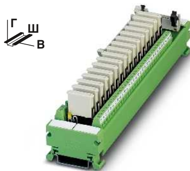
Базовый модуль вывода с 16 миниатюрными реле, 1 замыкающих контакта
