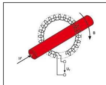
Определение действительного эффективного значения (TRMS) по принципу Роговского
