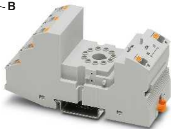
Базовый модуль для оконтального реле с тремя переключающими контактами
