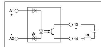
Рис. 3: 2-проводной выход
