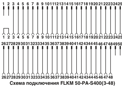
Схема подключения FLKM 50-PA-S400(3-48)
