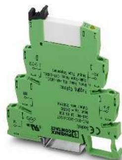
1 замыкающий контакт с силовым контактом
