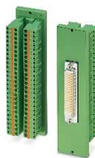
Со штыревой контактной частью разъема D-SUB и зажимом Push-in
