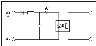
Рис. 1: Схема подключения, вход постоянного тока
