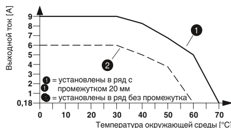
Кривая ухудшения характеристик ELR H5-SC-230AC/500AC-9. Продолжительность включения 100 %
