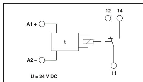
Реле времени с функцией попеременного включения, подача сигнала в начале импульса
