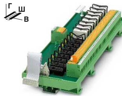
Модуль вывода и расширения для 16 мини-реле с клеммами с размыкателями, 1 переключающий контакт
