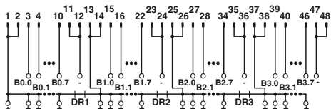
Схема подключения FLKM 50/32P/PLC
