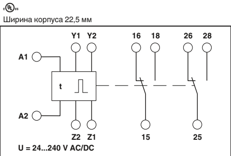
Многофункциональное реле времени, с двумя настройками времени
