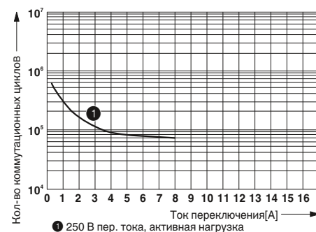
Срок службы электрического устройства
