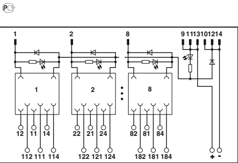
Модуль вывода для 8 миниатюрных реле, 2 переключающих контакта
