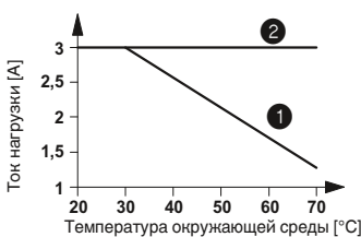
Кривая изменения характеристик для PLC-OSP...24DC/3RW
