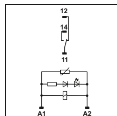
Катушка перемен. тока
