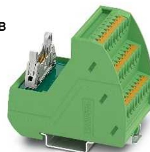
Модули инициатора с зажимами Push-in
