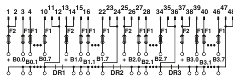
Схема подключения FLKM 50/32M/SI/PLC
