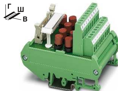
Пассивные модули с предохранителями для 8 или 32 каналов
