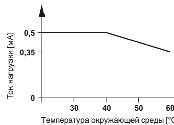
Кривая изменения характеристик PLC...24DC/48DC/500/W
