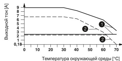
Кривая изменения характеристик ELR H3-IES-SC-24DC/500AC-2 и ELR H3-IES-SC-24DC/500AC-9 Продолжительность включения 100 %
