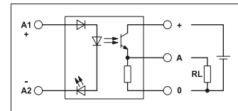
Рис. 4: 3-проводной выход
