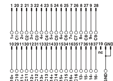
Схема подключения VIP-2/.../D37SUB/M/HW/C300
