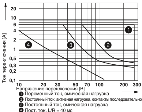
Электрическая мощность отключения для PLC...1IC/ACT для высоких пусковых токов
