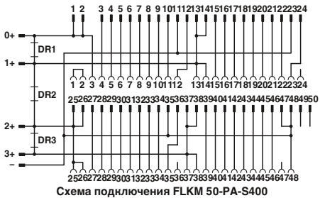
Схема подключения FLKM 50-PA-S400
