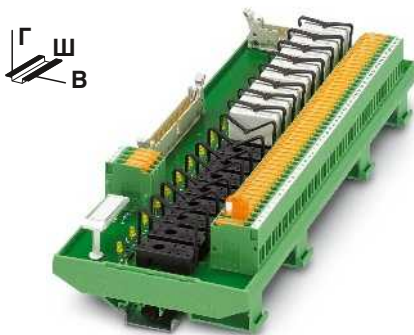
Модуль вывода для 16 мини-реле с клеммами с размыкателями, 1 переключающий контакт
