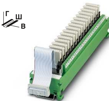
Модуль вывода и расширения с 16 миниатюрными реле, 1 замыкающий контакт
