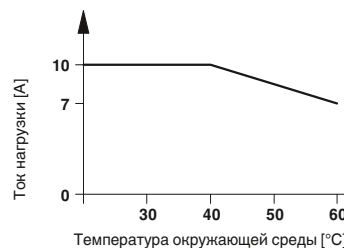
Кривая изменения характеристик для PLC-...24DC/24DC/10/R
