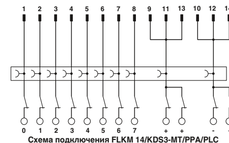
Схема подключения FLKM 14/KDS3-MT/PPA/PLC
