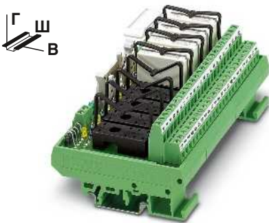
Модуль вывода для 8 миниатюрных реле, 2 переключающих контакта
