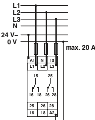
Пример подключения
