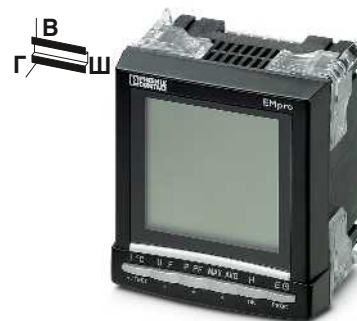
Измеряемое напряжение до 700 В переменного тока, с возможностью расширения
