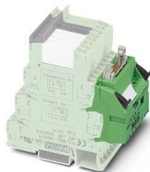
Адаптер VARIOFACE для модулей PLC (6,2 мм)
