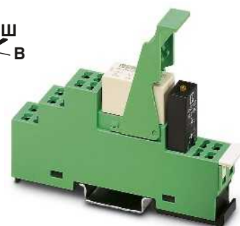
Релейный модуль PR1 с 1 переключающим контактом
