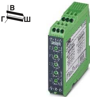
Реле контроля пониженного напряжения и фаз на 400 или 230 В
