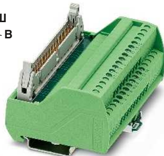
Соединительный модуль VARIOFACE для 16 каналов с винтовыми зажимами
