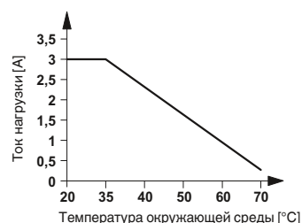
Кривая изменения характеристик для PLC-OSP...110DC/3RW
