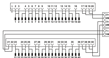
Схема подключения FLKM 50-PA/DO326/S7-S300
