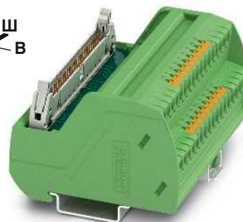
Соединительный модуль VARIOFACE для 16 каналов с зажимами Push-in
