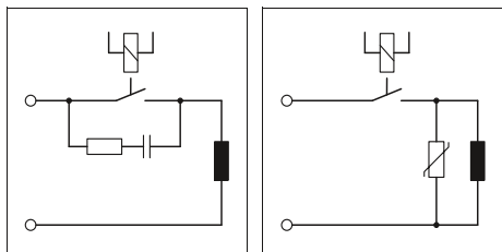
Схема подключена к контактам
