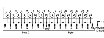
Схема подключения FLKM-PA-2D15/HW/DO/C300
