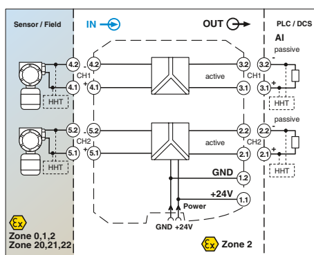
2-канальный барьер искрозащиты с питанием датчиков
