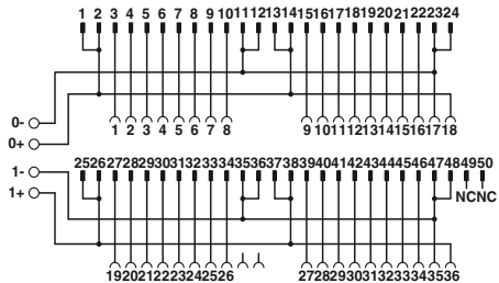
Схема подключения FLKM 50-PA-AB/1756/EXTC
