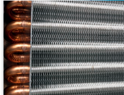
Большое расстояние между ламелями конденсатора
