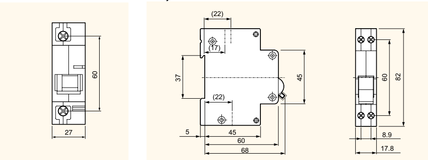
Рисунок 4 : Тип BKP
