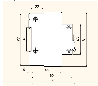
Рисунок 3 : Тип BKN
