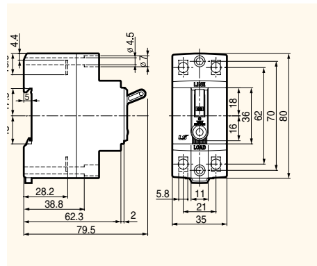
Рисунок 7 : Тип RKN-b
