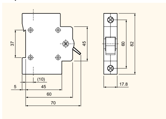
Рисунок 8 : Тип BKD
