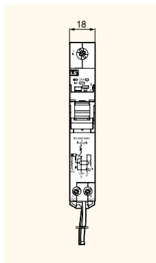
Рисунок 3 : Тип RKS-b
