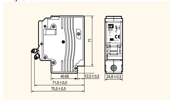
Рисунок 5 : Тип BFN
