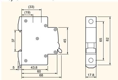
Рисунок 2 : Тип BKN-b
