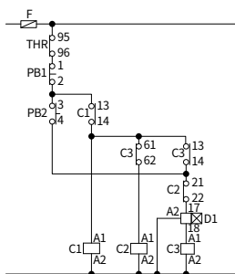
Схема подключения 1 (HGC9 ~ 100)
