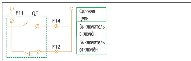
Схема подключения
