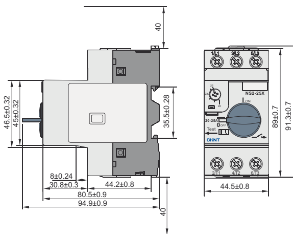
NS2-MC
