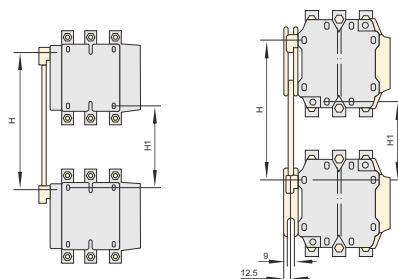
a. NC2-115Nc~225Nc
