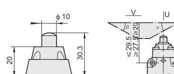
YBLX-P1/100/C YBLX-P1/120/C
