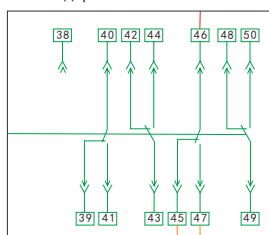
Модель схемы вспомогательных контактов
