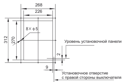
Размеры отверстия в оперативной панели
