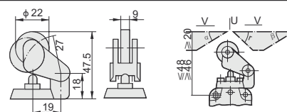
YBLX-P1/100/E YBLX-P1/120/E
