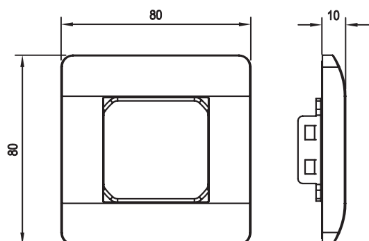
Рамка 1-постовая
