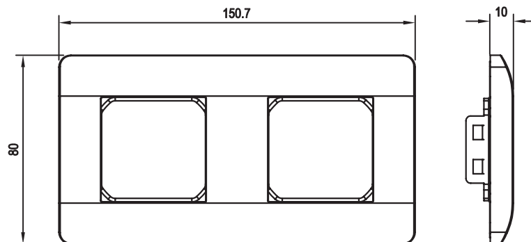
Рамка 2-постовая
