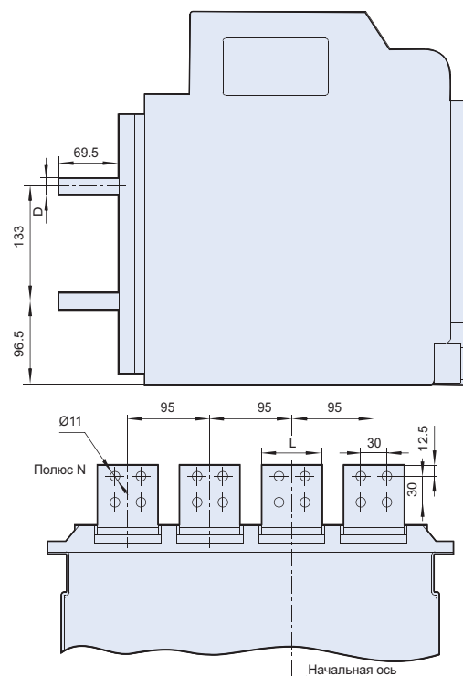
Размеры присоединяемых шин
