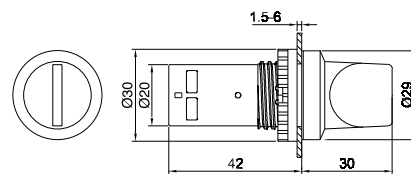
Переключатель
