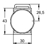
Джойстик
