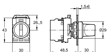
Переключатель
