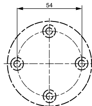
Схема сверления отверстий для сигнальных стоек K70
