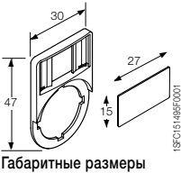
Габаритные размеры
