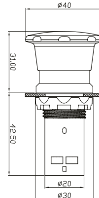
Грибовидная кнопка
