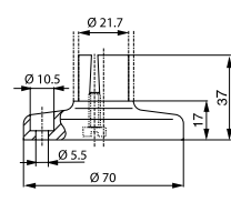
Звуковой модуль
