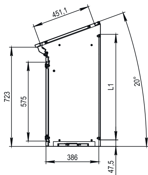
A-A (1 : 16)
