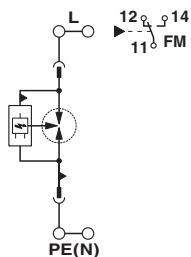
Электрическая схема
