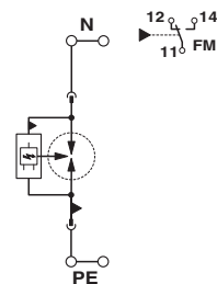
Электрическая схема
